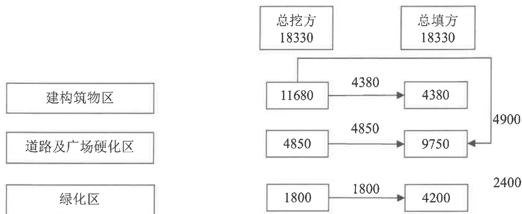
图 1.4-1 土石方流向图 单位：m 3
