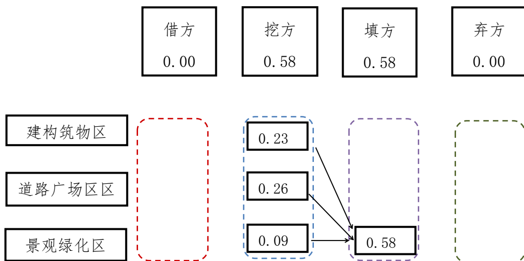
图1 本项目表土平衡流向框图 单位：万 m 3
