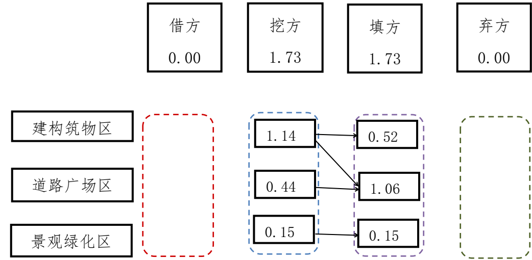
图2 本项目主体工程建设土石方平衡流向框图 单位：万 m 3
