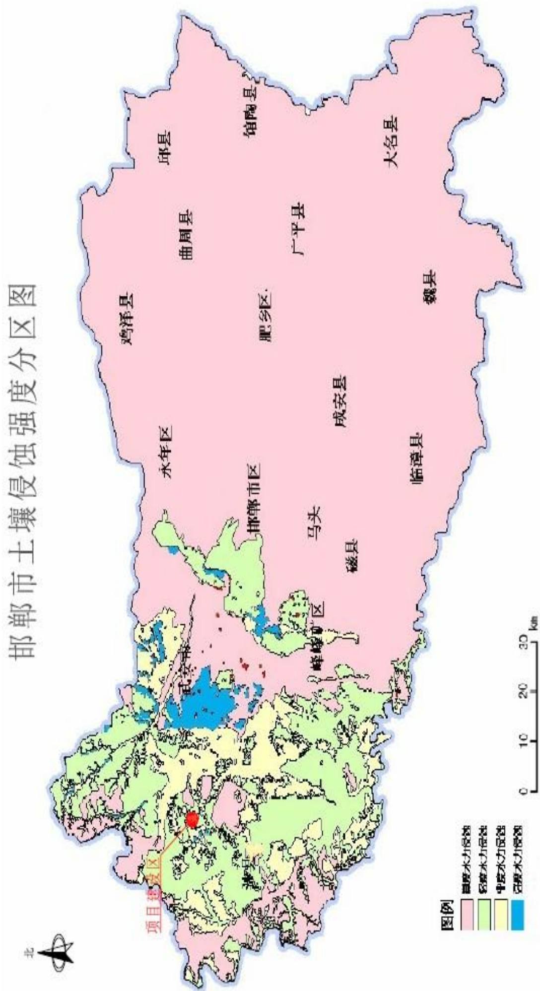
附图3：项目区土壤侵蚀图
